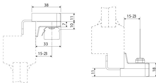
Кронштейн накладной металлический (2 типоразмера)
